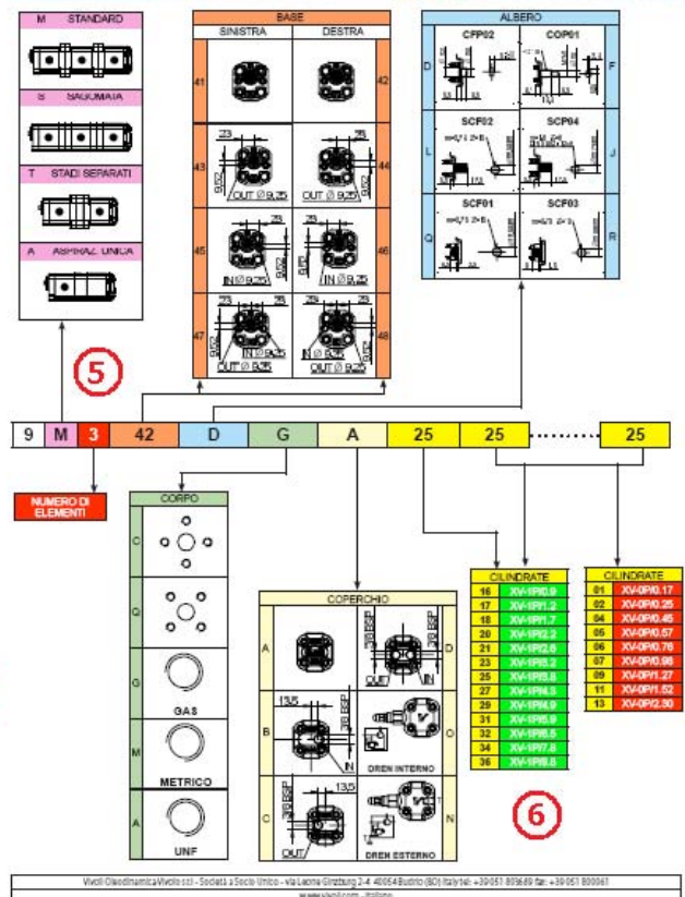
POMPA MULTIPLA XV-1 BASE ø 32 Sagomata - TIPO "BH"
